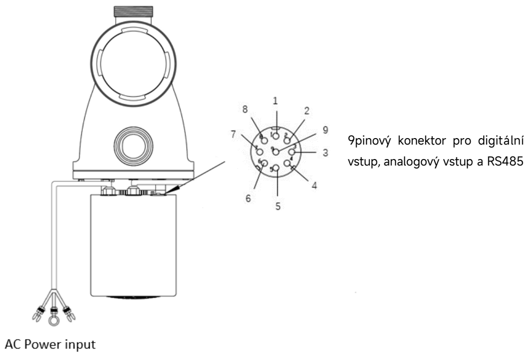
Obrázek 6 - Digitální vstup, Analogový vstup a konektor RS485
