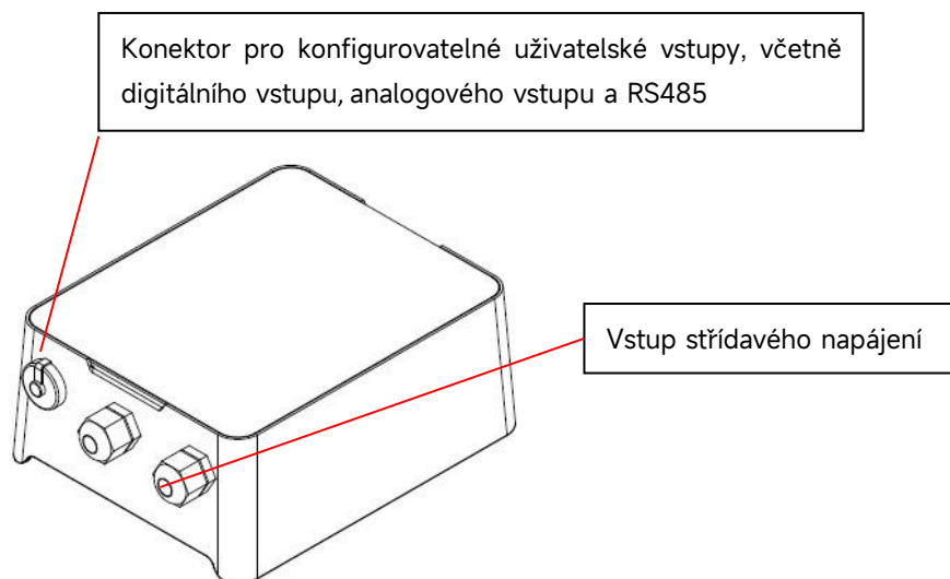
Obrázek 5 - Umístění portu konektoru
