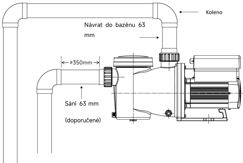
Obrázek 2 - Instalace vodovodního potrubí a armatur
