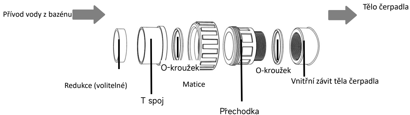
Obrázek 3 - Sada pro připojení
