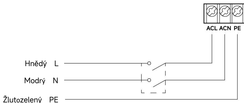
Obrázek 7 - Připojení napájecího kabelu
