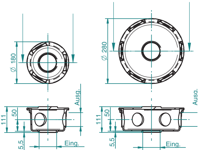
Wasserverteiler ø150mm Art.-Nr.: 4824050 Art.-Nr.: 4824150 Art.-Nr.: 4824250 Wasserverteiler ø250mm Art.-Nr.: 4825350 Art.-Nr.: 4825450 Art.-Nr.: 4825550
