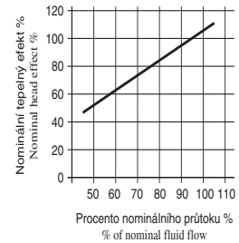
Korekce průtoku, Correction Factors teplota, průtok, Temperature and Flow Rate, diagram B
