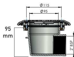
4827814 s mosaznými zástříky 4827814 with brass inserts
